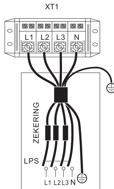
VOEDING VAN BINNENUNIT 3-fasige 3/6/9 kW back-upverwarming
