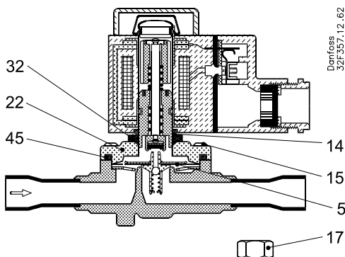
EVRC 10 and 15 (NO)
