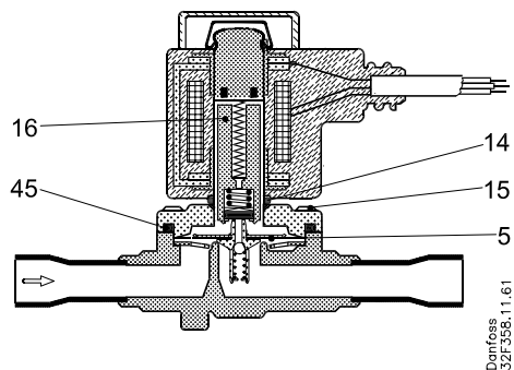
EVRC 10 and 15 (NC)
